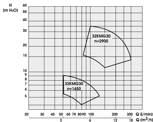
Wykres pracy pomp KGM KMG pump operation diagram
